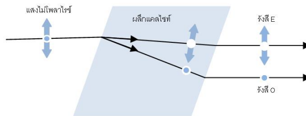
การหักเหสองแนวเมื่อแสงไมโพลารไรซ์ผ่านผลึกแคลไซต์
